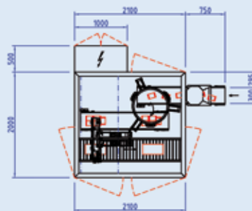
Grundriss (M 1:100)
