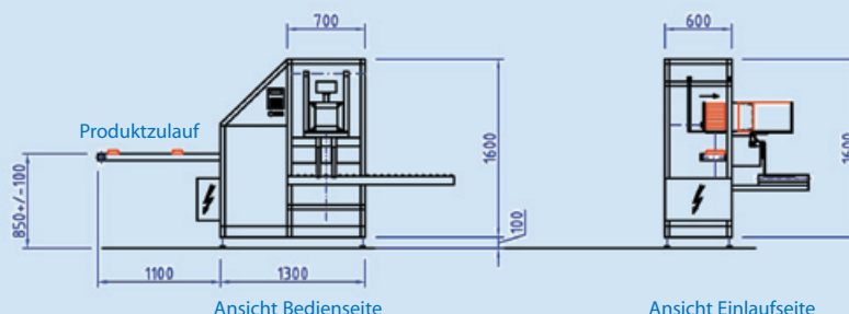
Ansicht Einlaufseite
